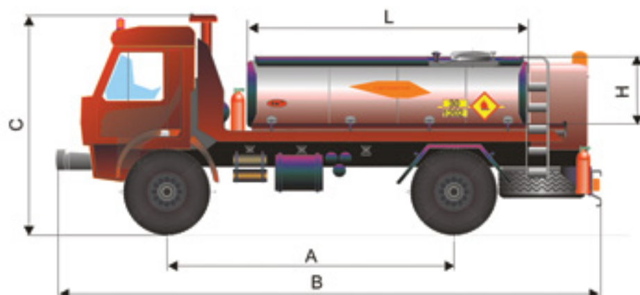
AUTOCISTERNE ZA PREVOZ GORIVA OD 6000 DO 16000 L
