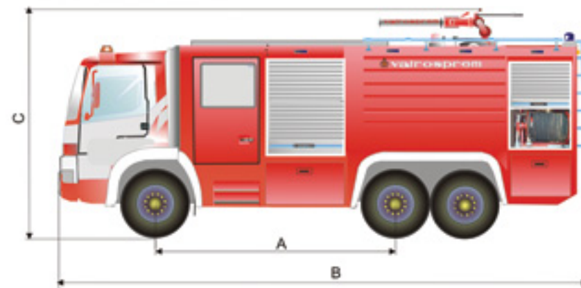
VATROGASNA VOZILA ZA GAŠENJE VODOM KAPACITETA OD 3000 DO 14000 L
